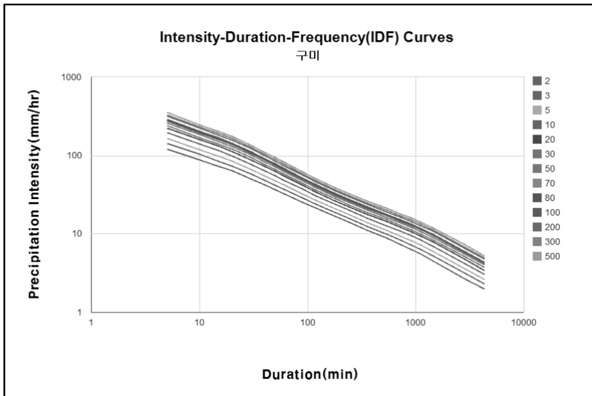
【그림 12.8】 구미지역 IDF곡선
